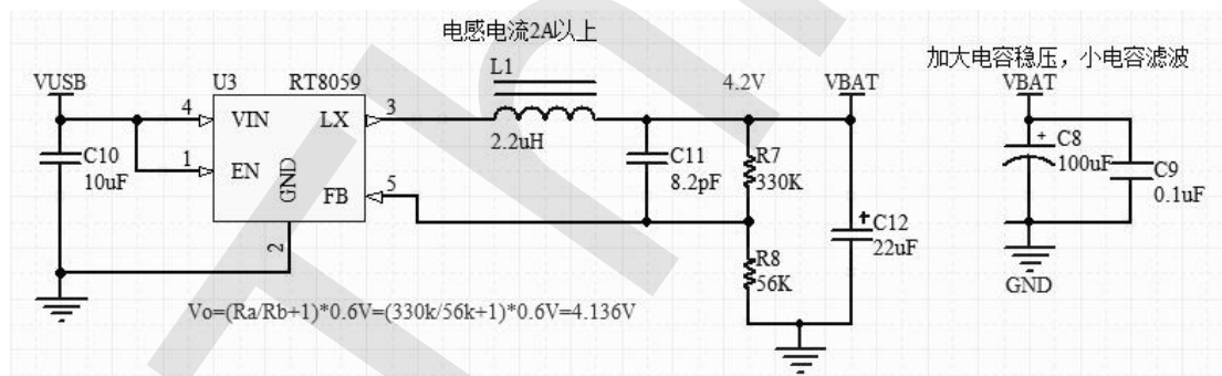
图 4.2 A9 电源供电电路
