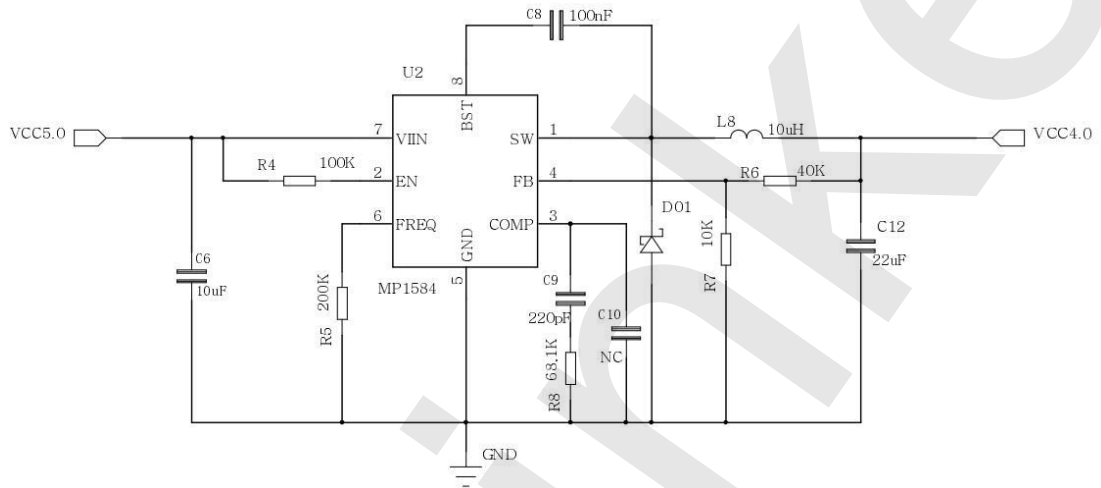
图 4.1 A6 供电电路参考设计
