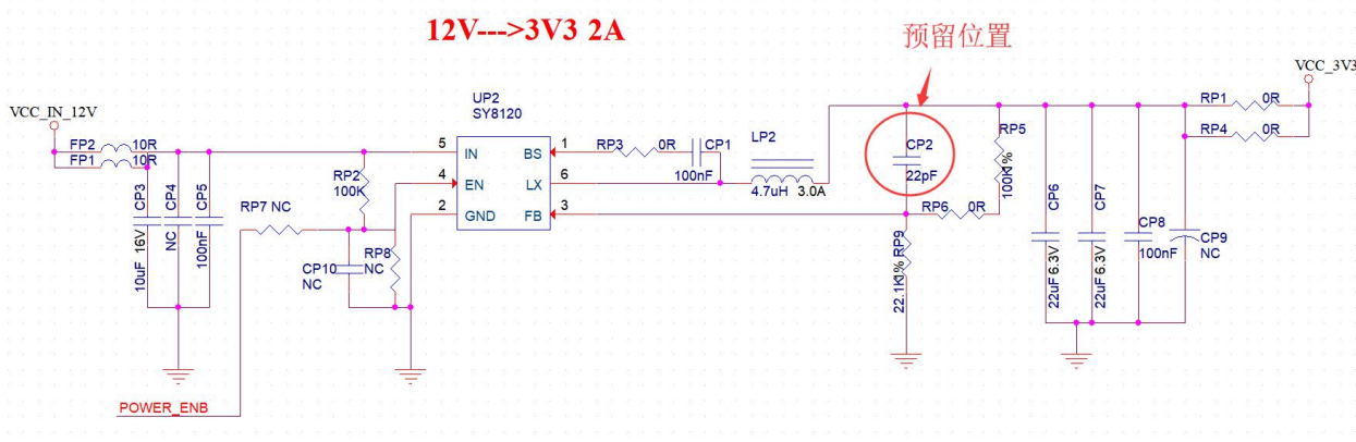
图 9 DC-DC 降压电路图
