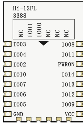
图 5 管脚示意图
