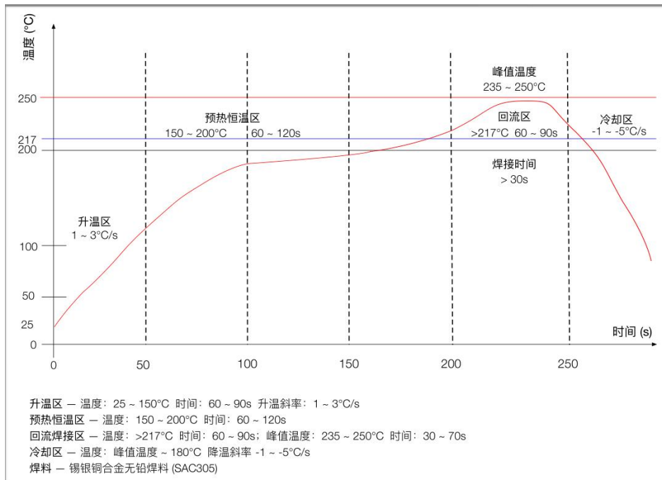
图 11 回流焊曲线图
