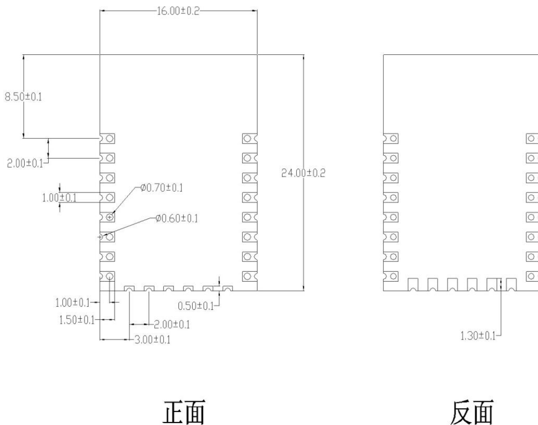
图 4 模组尺寸图
