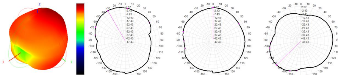
960M 3D-E1-E2-H
