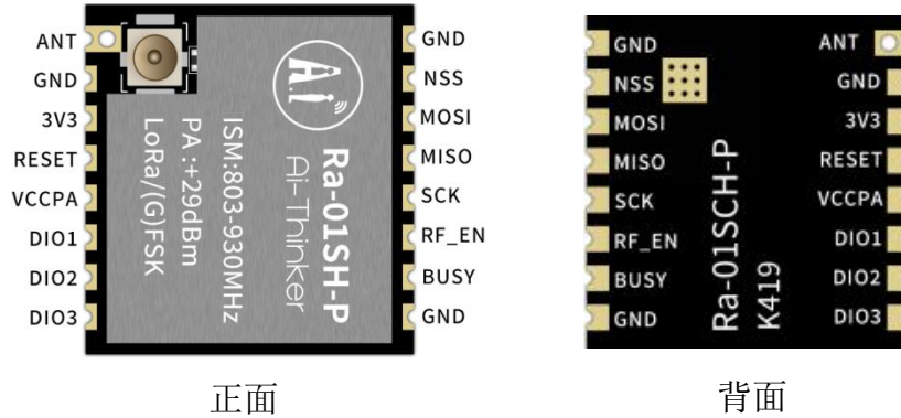
图 5 管脚示意图
