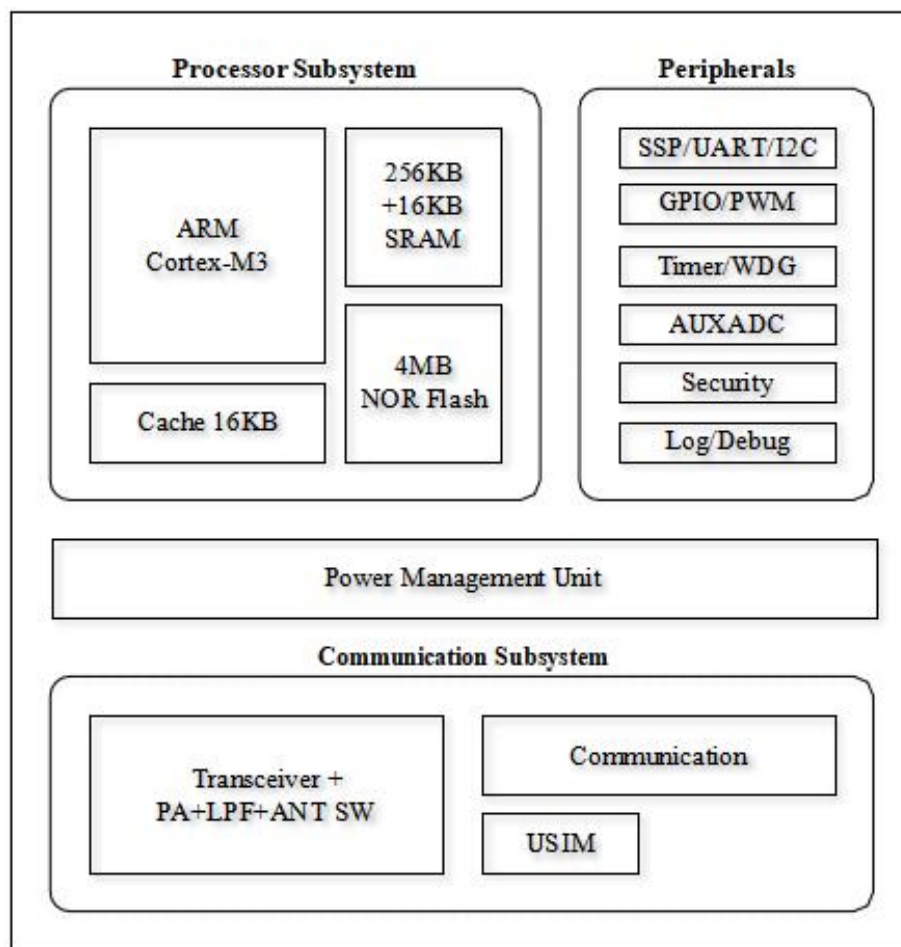
图 1 芯片架构图
