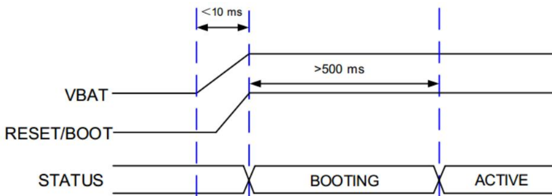
图 10 NB 芯片上电时序图
