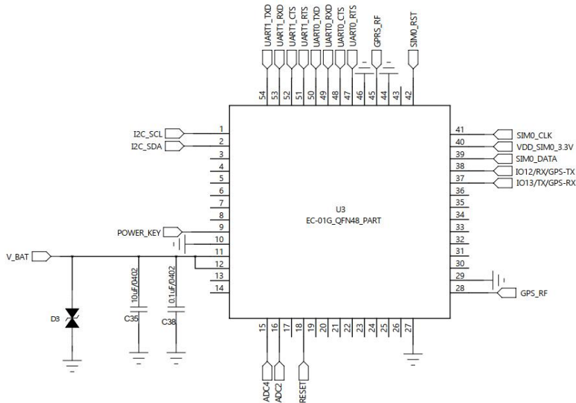
图 8 应用电路原理图
