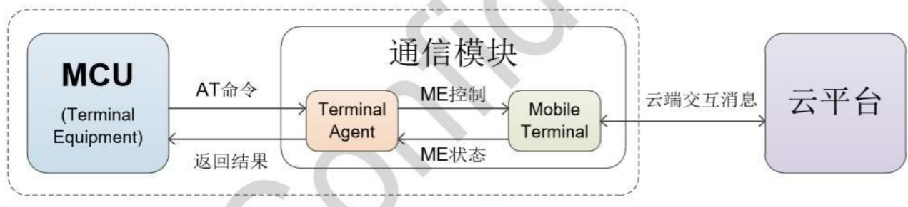
图 1-1 系统结构图
