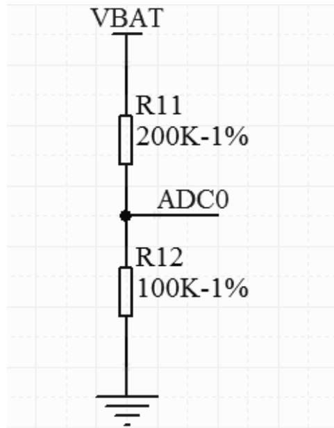
图 4.8 A9 ADC 设计参考图
