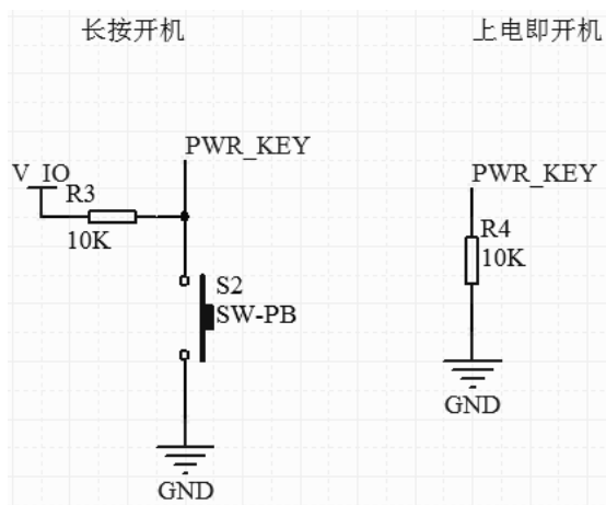
图 4.4 开关机电路参考设计
