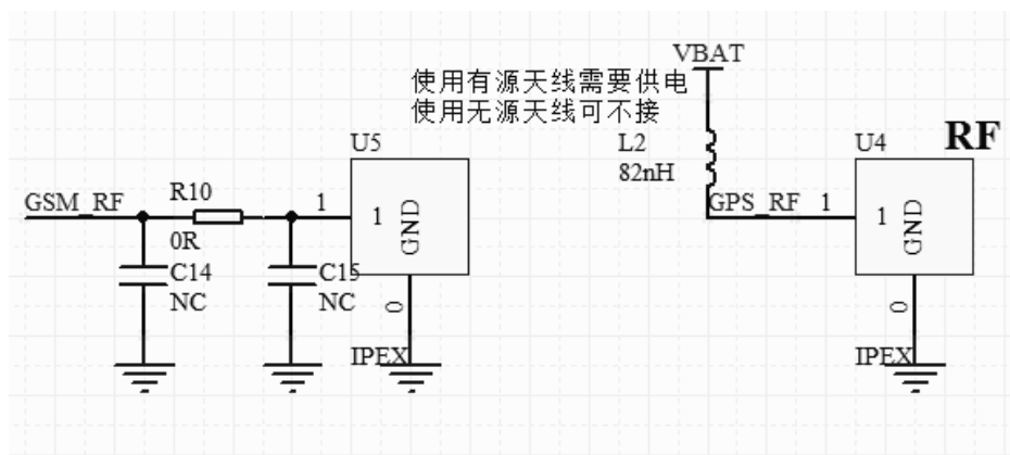
图 4.11 天线参考设计
