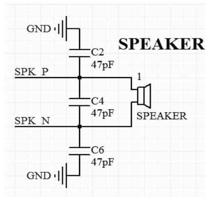
图 4.9 SPEAKER 参考设计
