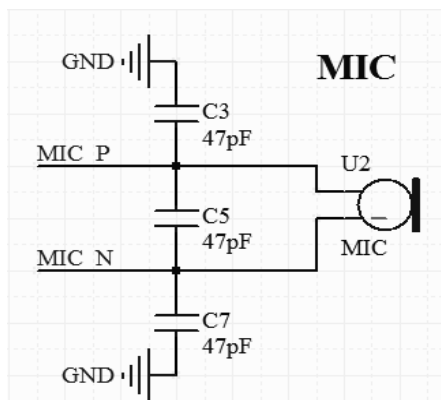
图 4.10 MIC 参考设计
