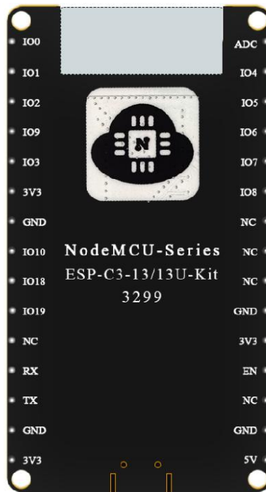
ESP-C3-13-Kit 管脚示意图
