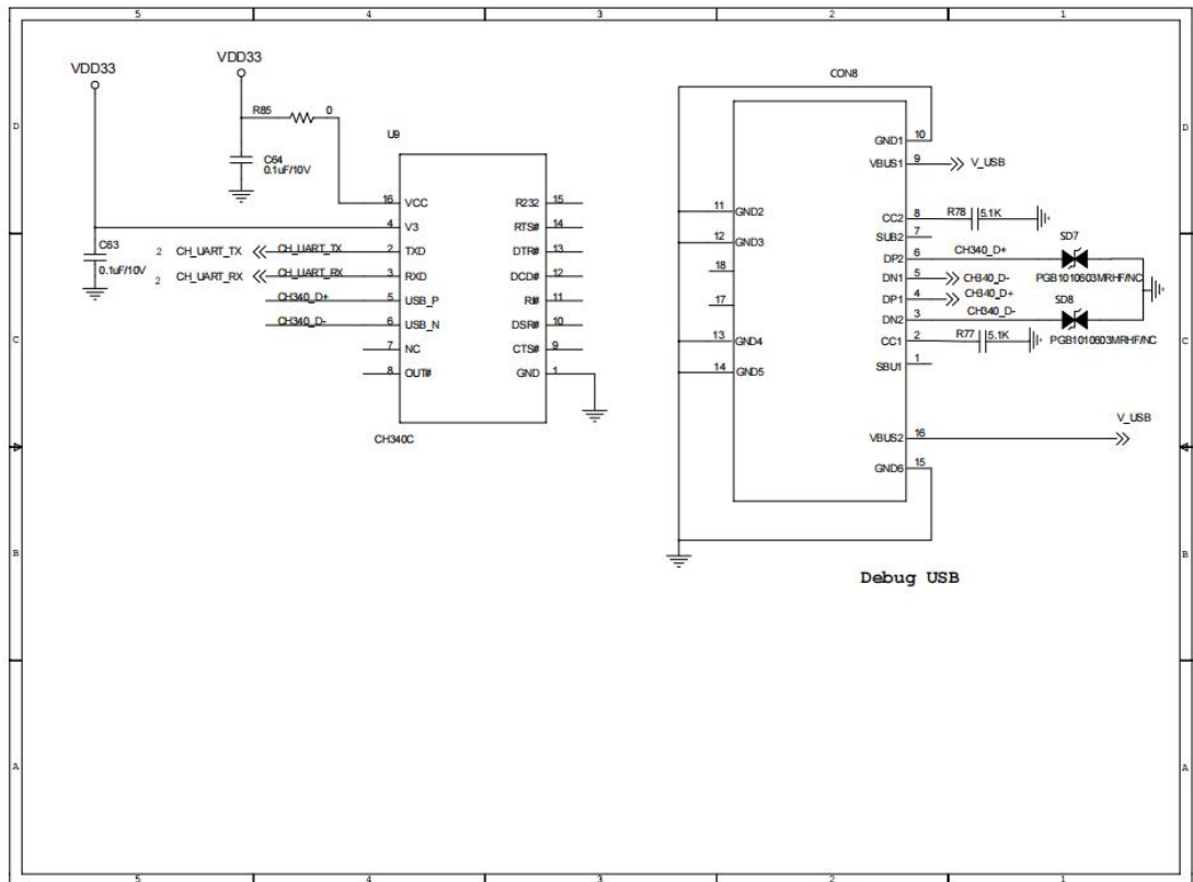
图 7 开发板原理图
