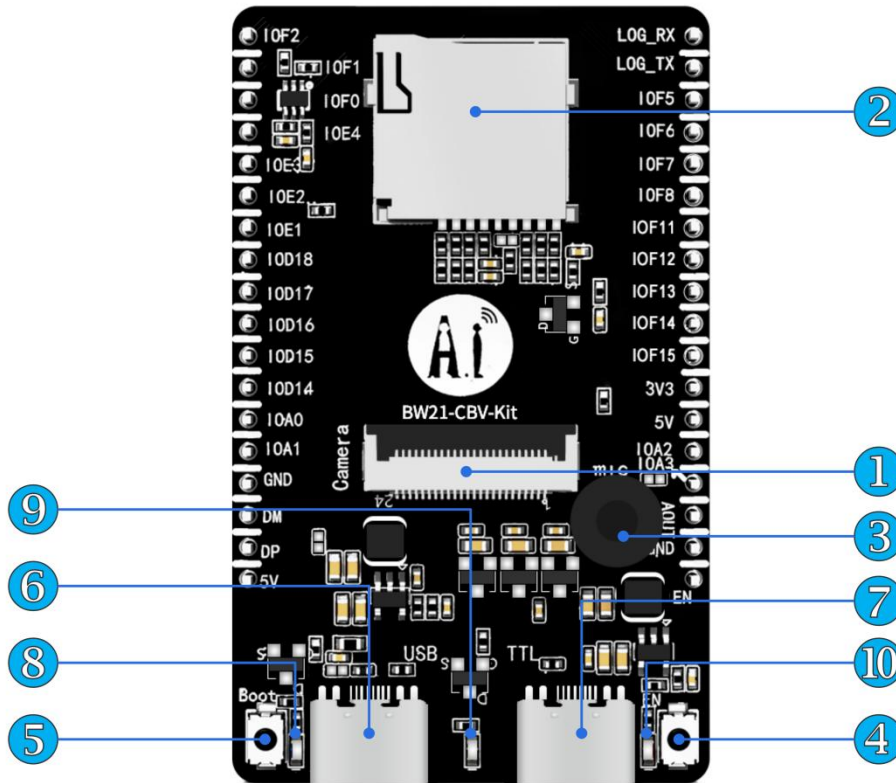
图 5 接口指示图
