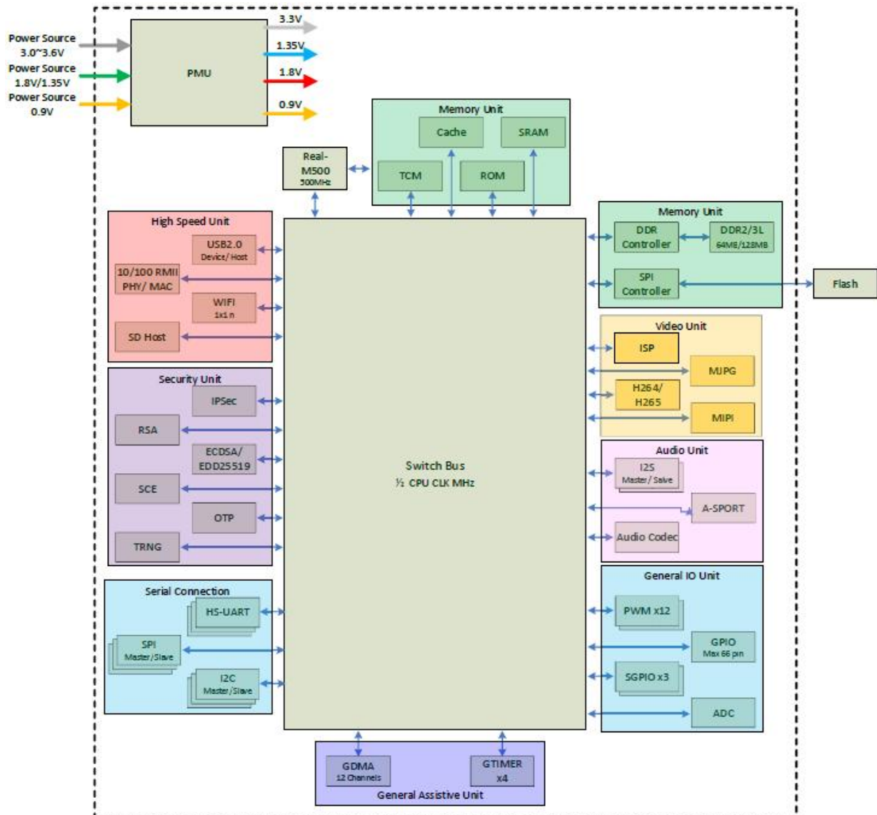
图 1 主芯片架构图
