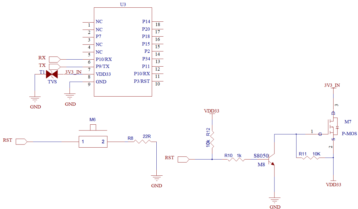
图 10 应用电路图
