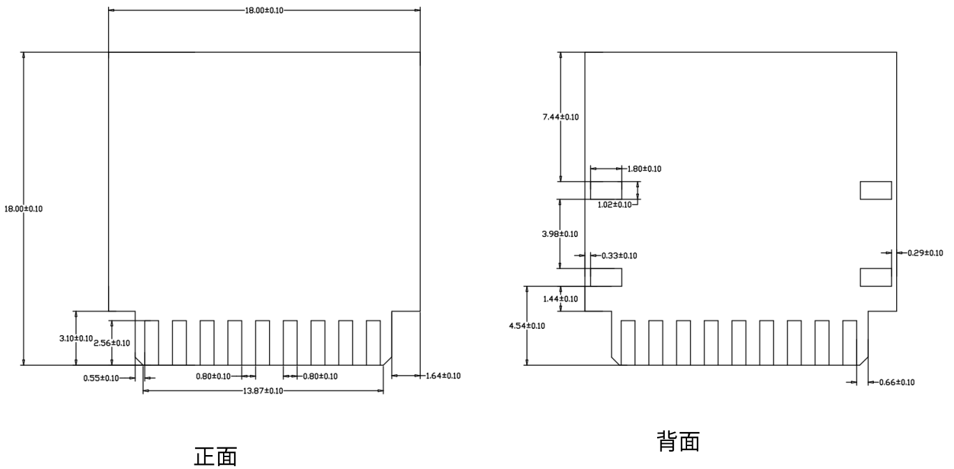
图 4 模组尺寸图
