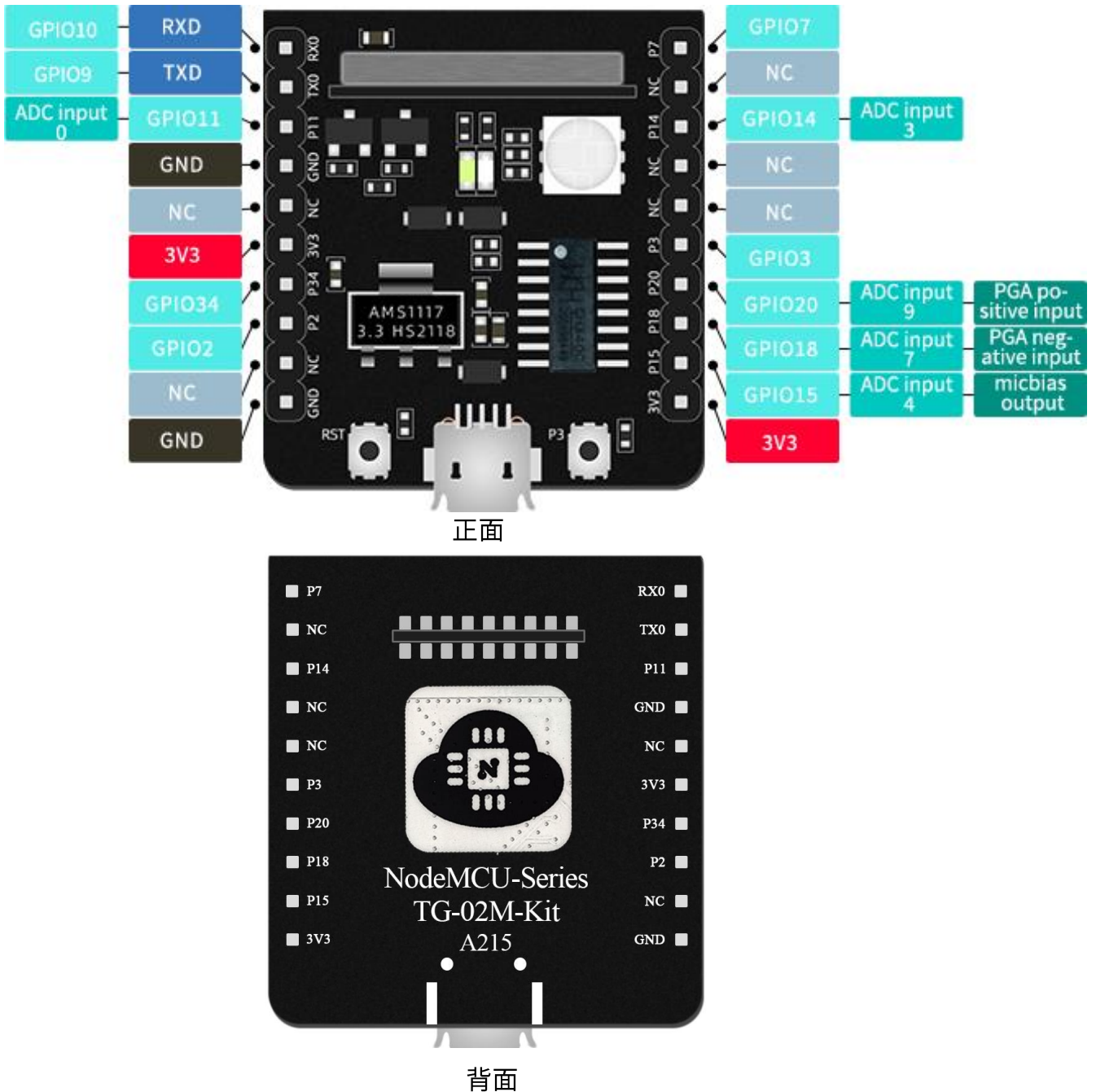
图 6 开发板管脚示意图
