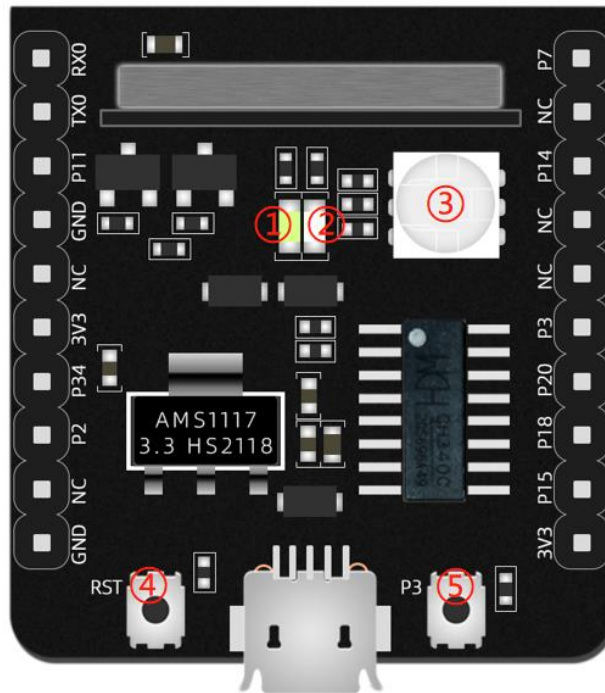
图 5 TG-02M-Kit 指示灯及按键位置
