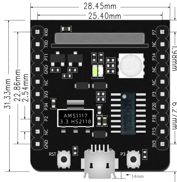
图 4 开发板尺寸图
