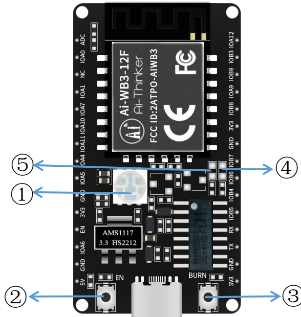
图 5 Ai-WB3-12F-Kit 指示灯及按键位置
