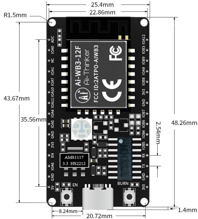
图 4 尺寸图
