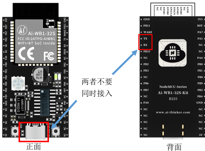
图 8 接口示意图
