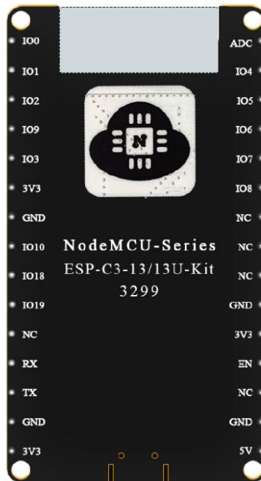
ESP-C3-13U-Kit 管脚示意图
